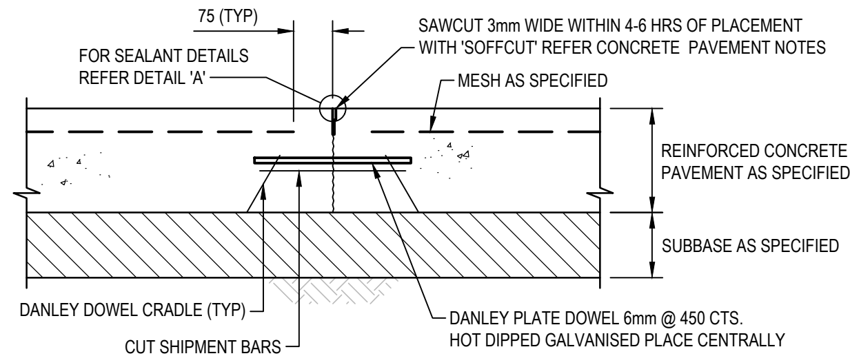
SAWCUT JOINT (SJ) (POUR OVER) SCALE 1:10
